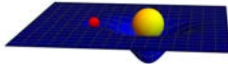
FIGURA 2. Relatividade Geral: o espaço-tempo é curvado por objetos com massa.
