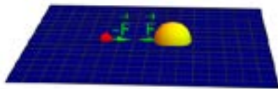
FIGURA 1. Teoria da gravitação de Newton: forças gravitacionais.
