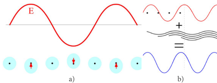
Figura 1 (a) O campo elétrico da onda que está a atravessar o material provoca uma oscilação da nuvem eletrónica dos átomos, ou moléculas, dando origem a um dipolo elétrico. (b) Cada dipolo elétrico em oscilação vai dar origem a uma nova onda eletromagnética. Estas ondas secundárias estão normalmente atrasadas em fase relativamente à onda inicial. A soma das ondas secundárias com a original dá origem a uma onda que parece viajar mais lentamente pela presença da matéria.
