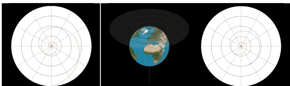
FIGURA 2. Comparação da espiral logarítmica, à esquerda, com a espiral de Poincaré, à direita, correspondentes, respetivamente, às projeções estereográfica e ortográfica de uma loxodromia com azimute de 76^\circ .
