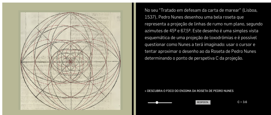
FIGURA 3. As espirais sobrepostas sobre os arcos de circunferência da roseta de Pedro Nunes esclarecem o enigma.
