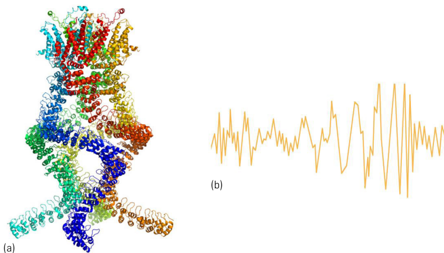
(a) Um sensor do tipo que lê as variações de pressão no ouvido e nos permite ouvir. (b) A primeira onda gravitacional detetada, mostrando a chegada do sinal resultante do colapso de dois buracos negros.
