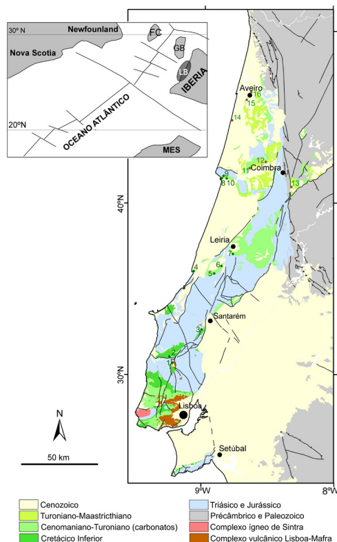
FIGURA 1. Localização geográfica das principais jazidas de mesofósseis: 1- Catefica, 2- Torres Vedras, 3- Cercal, 4- Nazaré, 5- Juncal, 6- Vale de Água, 7- Fomalicão, 8- Buarcos, 9- Tavarede, 10- Vila Verde, 11- Vila Verde de Tentugal, 12- Ançã, 13- Vila Flor, 14- Mira, 15- Presa, 16- Esgueira.
