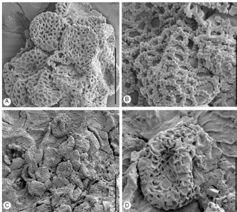
FIGURA 3. Imagens de microscopia eletrônica de varrimento de pólenes de angiospérmicas. A-B – Cluster de pólenes de tipo Pennipollis do Cretáceo Inferior de Torres Vedras. C-D – Grãos de pólen de tipo Retimonocolpites do Cretáceo Inferior do Juncal. Escala: A – 20 µm; B – 10 µm; C – 25 µm; D – 10 µm.
