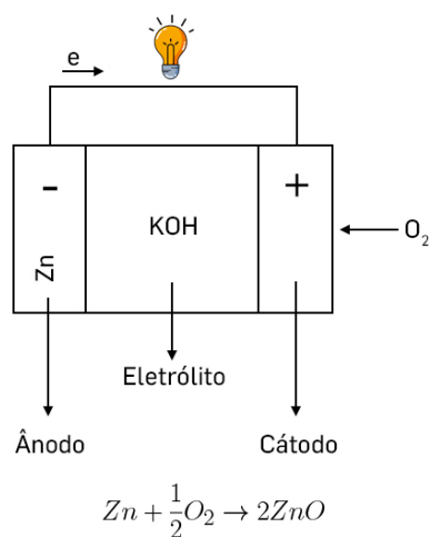
FIGURA 1. Célula eletroquímica zinco-ar primária.
